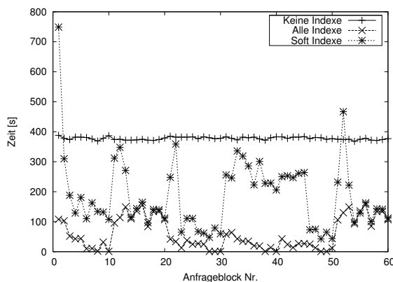
Abbildung 6: Adaptionverhalten
